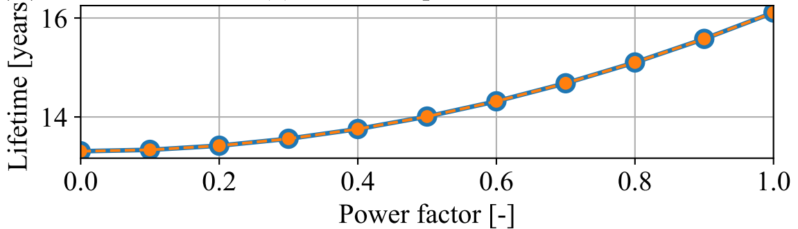
(d) DC-link capacitor lifetime
